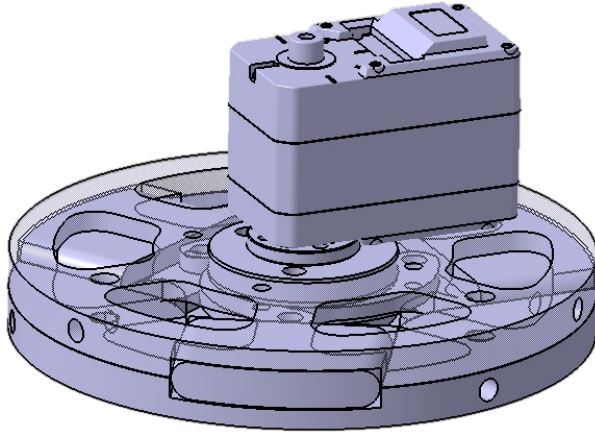
FIGURE 4.4 – Système d'aérofrein d'SP-02 sur CA-TIA
