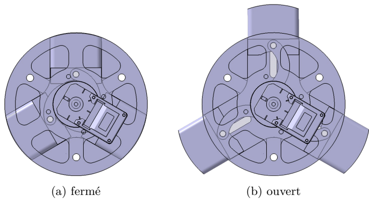
FIGURE 4.5 – Position des aérofreins d'SP-02
