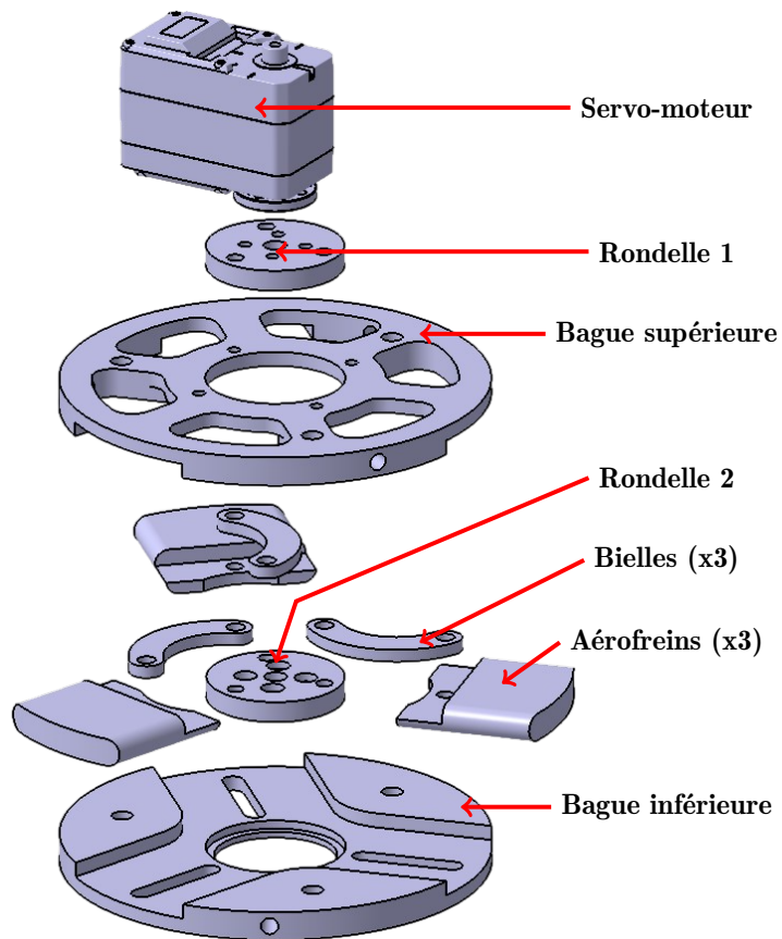
FIGURE 4.6 – Vu éclatée du système d'aérofrein d'SP-02
